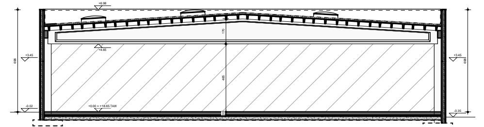
Principesnede AA schaal 1:250
